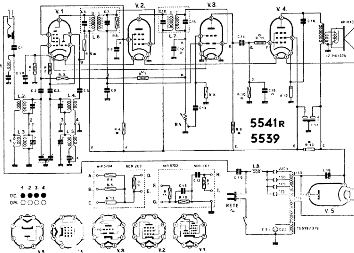
FIMI S. A. - PHONOLA - Modd. 5539, 5541 R e 5543 R Soprammobili. Onde medie da 185 a 576 m; onde corte da 18 a 52 m. Media frequenza 470 KHz. Consumo 35 watt. Potenza indistorta 3 watt.
